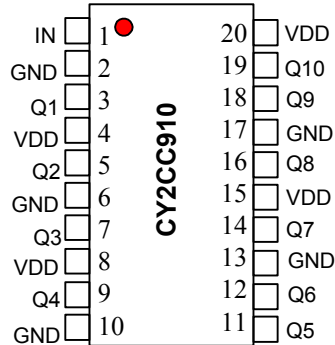
20 pin SOIC/SSOP
